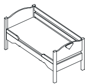
Кровать детская с ограждением (спальное место 140x70)
