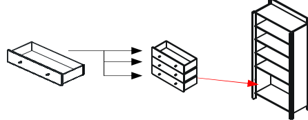
Ящик выдвигающей для установки в этажерку широкую 63ЭТ23 844x320xh590(196x3)
